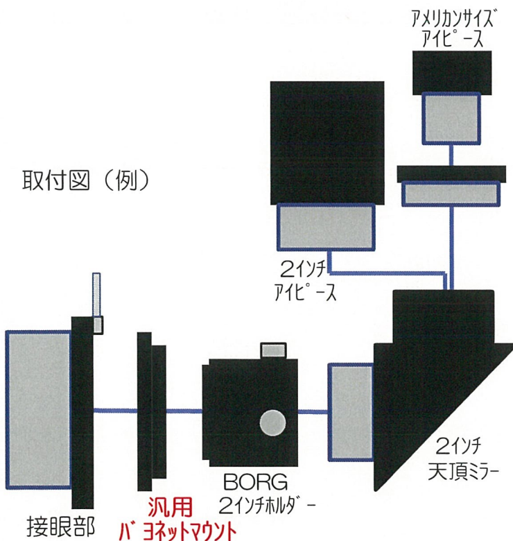
15cm屈折赤道儀2インチアクセサリ装着例
